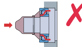
Montáž do tělesa s přesahem
