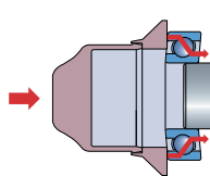
Montáž na hřídel s přesahem
